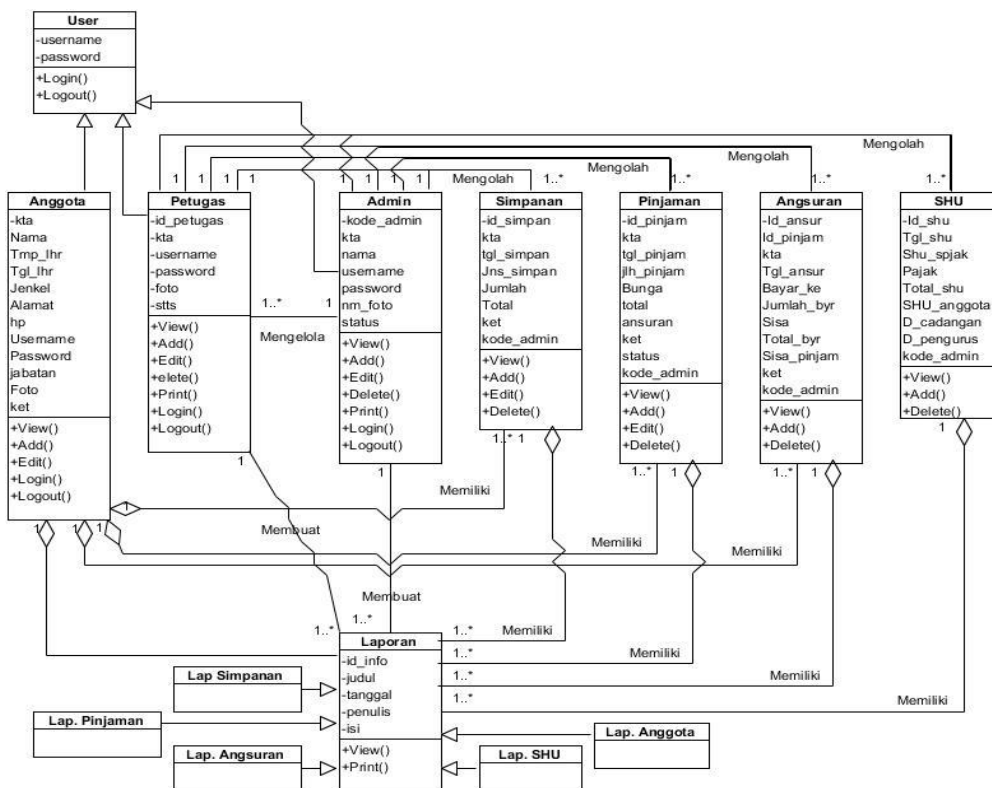
Gambar 12. Diagram Class Sistem Simpan Pinjam Koperasi Tanjung Sari
