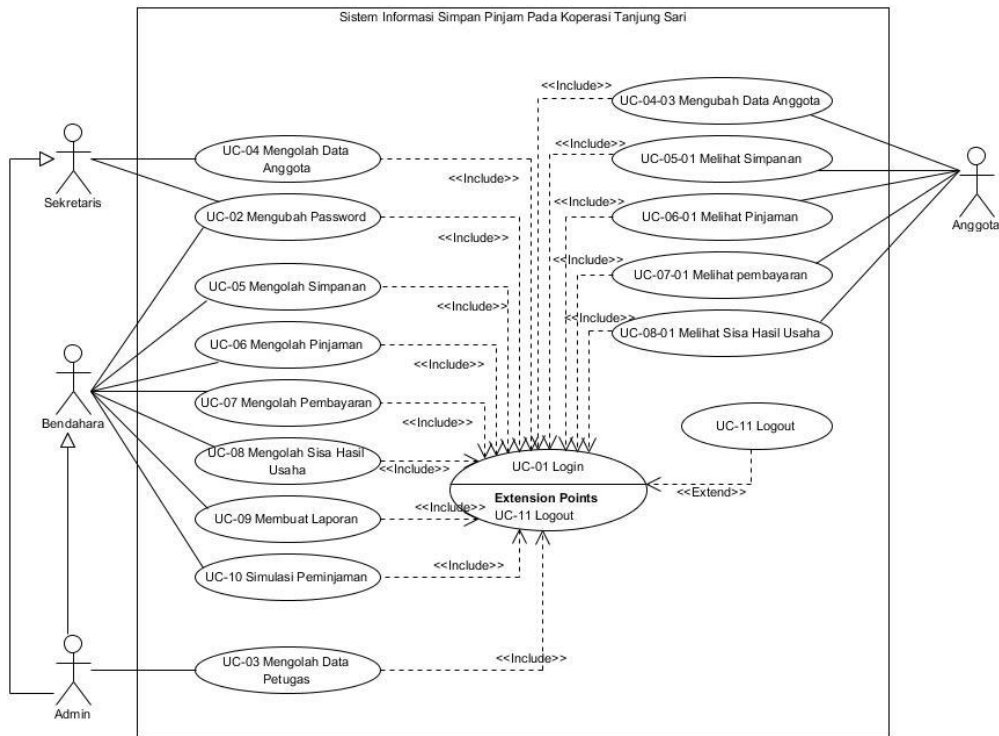
Gambar Diagram Use Case Sistem Informasi Simpan Pinjam Pada Koperasi Tanjung Sari
